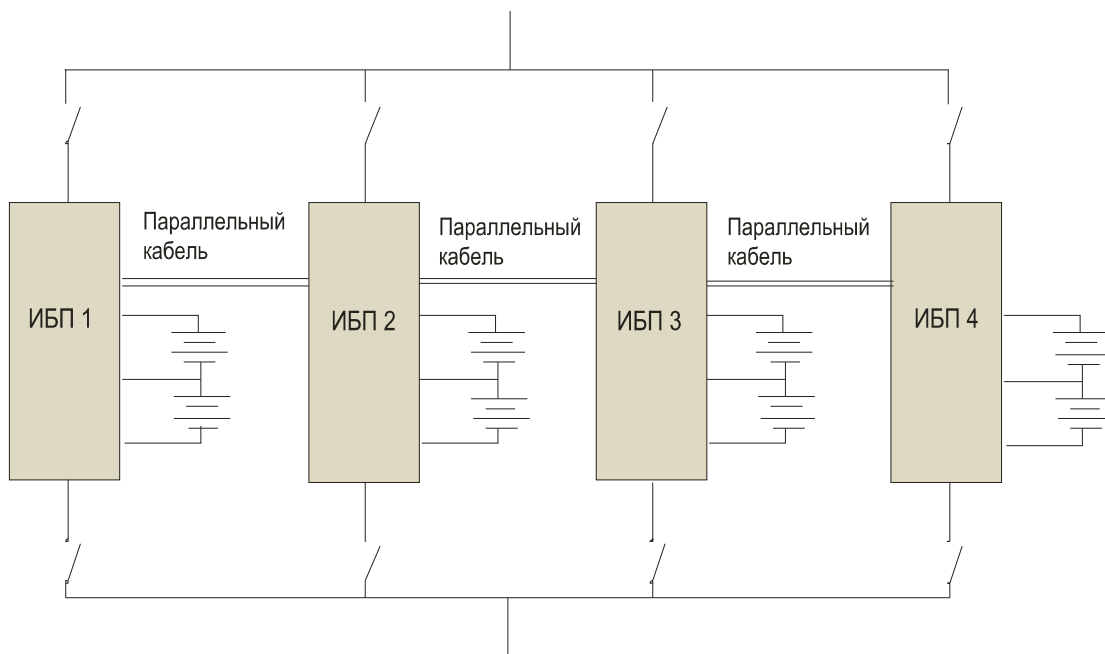
Рис.2-3 Параллельная система
