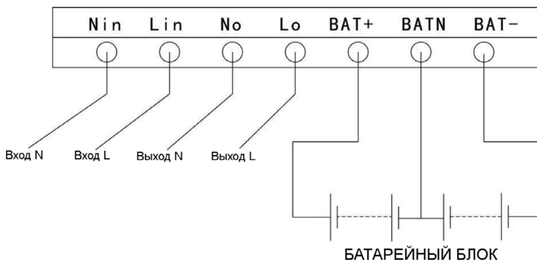
Рис. 2-2 Подключение к клеммной колодке
